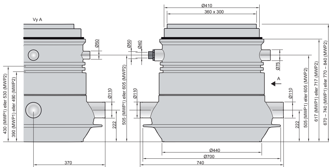
Bild 6: Måttfigurer
